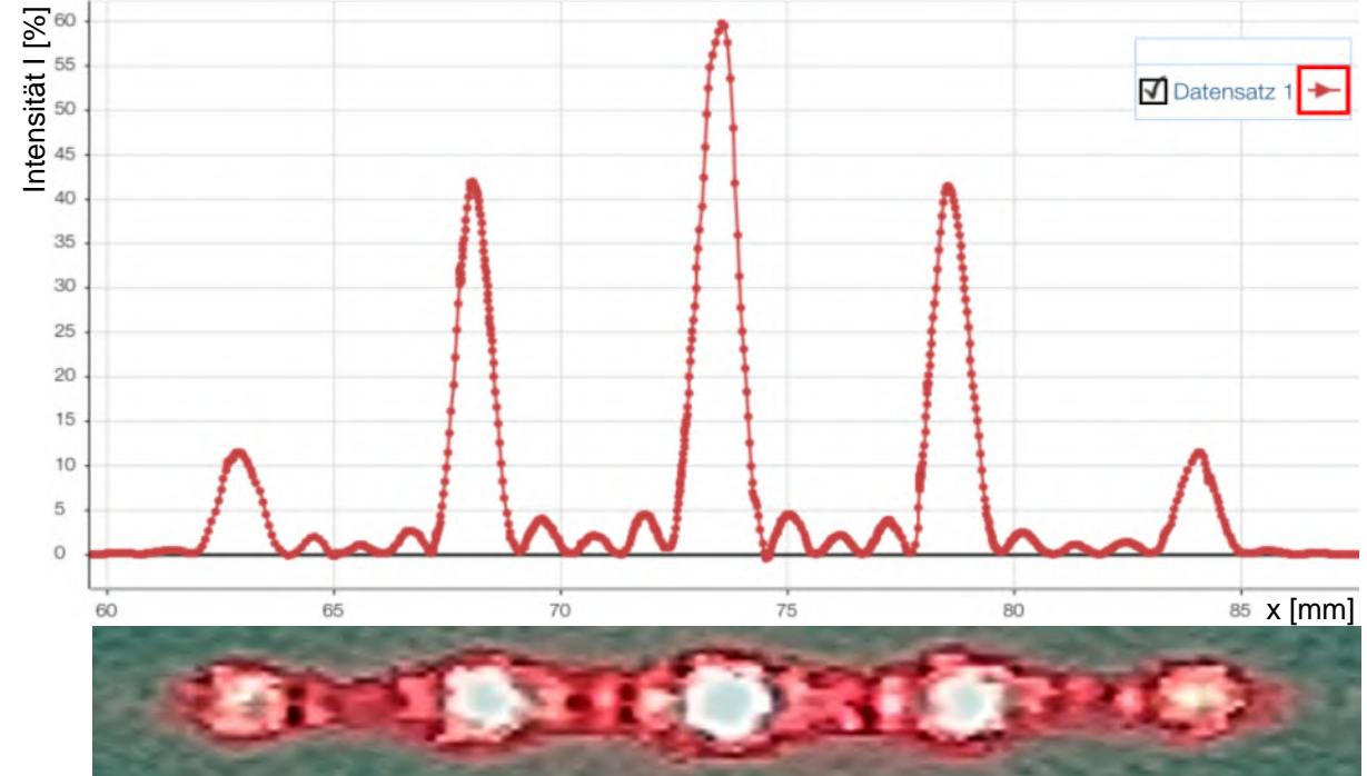
Firma Vernier: Diffraction Apparatus
