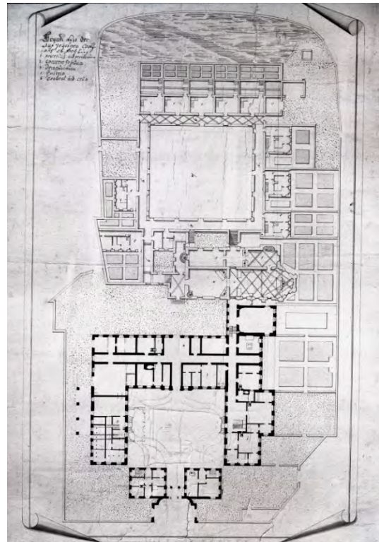
Abb. 2: Historischer Grundriss der Kartause, nach 1782. Auf dem Plan sind die heute nicht mehr erhaltenen Mönchszellen abgebildet. Stadtarchiv Freiburg, M 10/52. Foto: Frank Hack.
